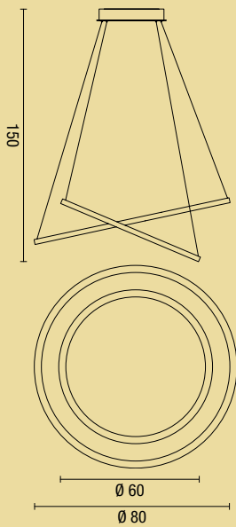
sospensione Aluring doppio anello Aluring double rings pendant lamp
